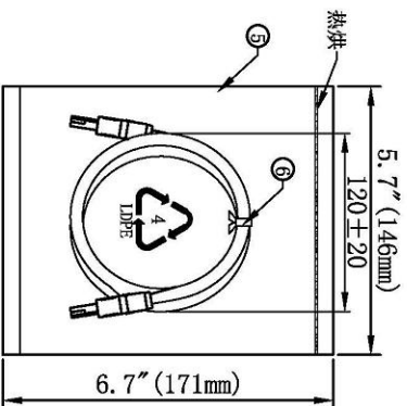
包装示意图
