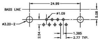
P.C.B. LAYOUT
