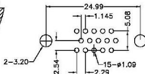
P.C.E. LAYOUT
